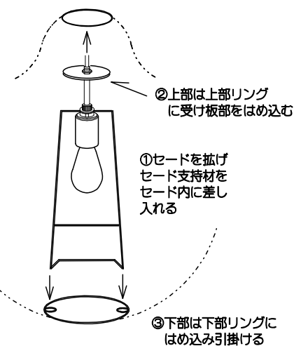
図2) セードの組立方法
