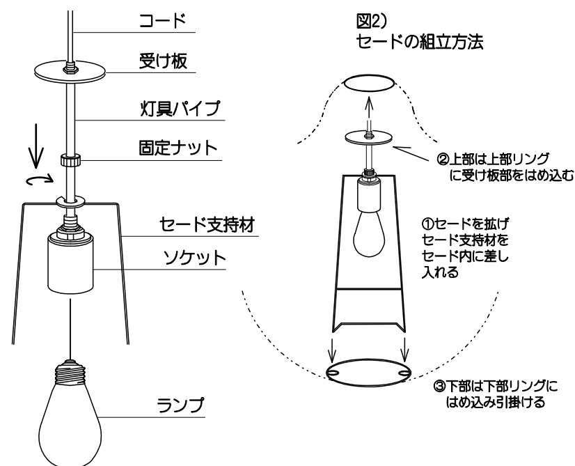
図1) 灯具とセード支持材の組立方法
