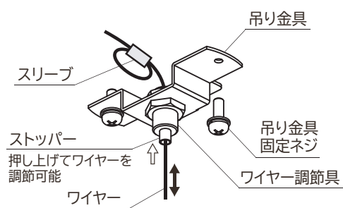
図1 ワイヤ吊金具
