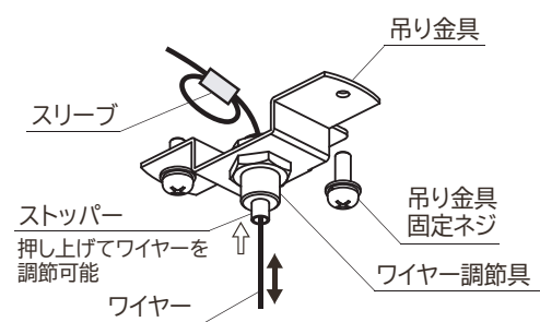
図1 ワイヤー吊金具
