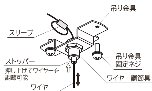
図1 ワイヤー吊金具
