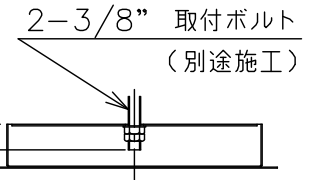
取付部詳細
