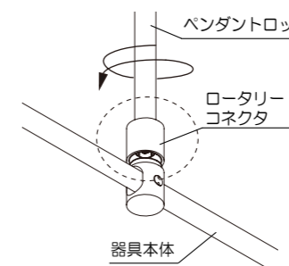
ペンダントロッド、器具本体端部を付属のロータリーコネクタでねじ込む。 ※ロータリーコネクタは個別にフリー回転します。コネクタのみをしっかりと回して電氣的に接続される状態にしてください。
