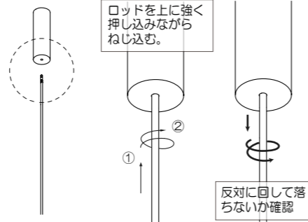
図6 ロッドをフランジに押し込みながら、しっかりとねじ込む。 ※ロッドは360°フリー回転なので、正しく取付されても回り続けます。組立後は下に引きながら反対に回し、ロッドが抜けかないか確認してください
