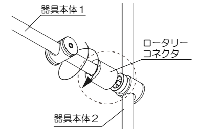
ペンダントロッド、器具本体端部を付属のロータリーコネクタでねじ込む。 ※ロータリーコネクタは個別にフリー回転します。コネクタのみをしっかりと回して電氣的に接続される状態にしてください。
