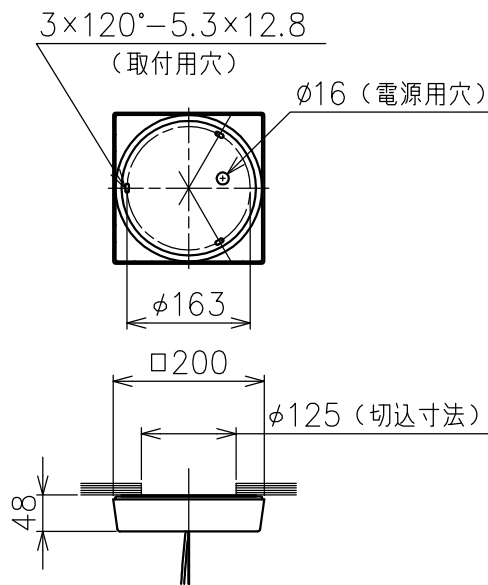
取付板部詳細 S:1/10
