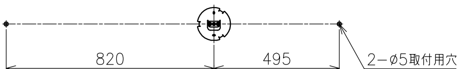
取付板詳細 S:1/5
