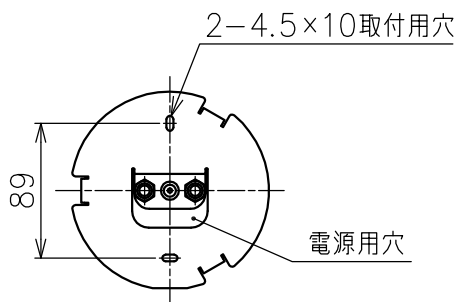
取付板詳細 S:1/5
