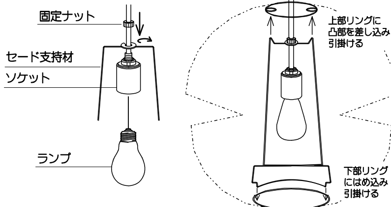
図2) 灯具とセード支持材の組立固定取付
