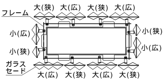
フレームにガラスセードを取付け、器具を上から見た図
