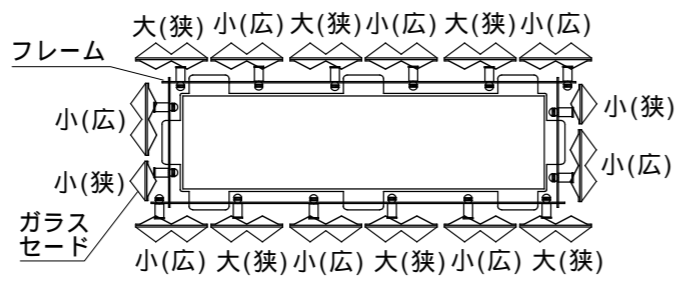
フレームにガラスセードを取付け、器具を上から見た図
