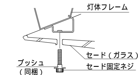
図1)セード(ガラス)固定方法 断面図
