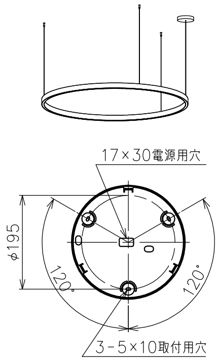
取付板詳細
