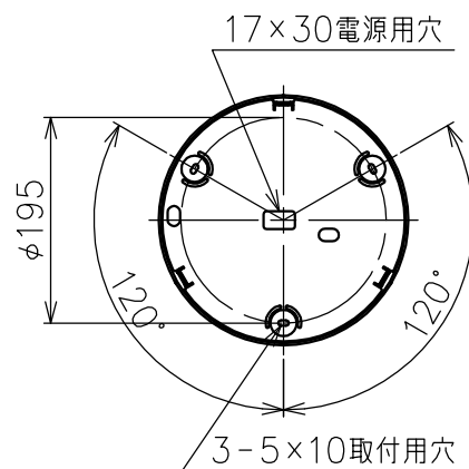
取付板詳細
