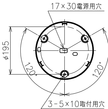
取付板詳細
