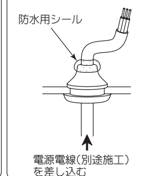
図5 電源電線防水処理
