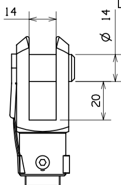
Detail beliere echelle 1:2
