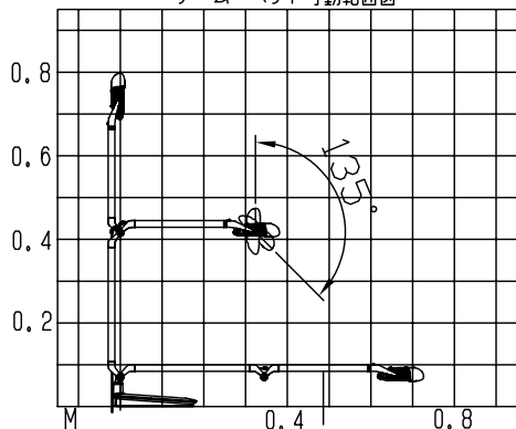
アーム・ヘッド可動範囲図
