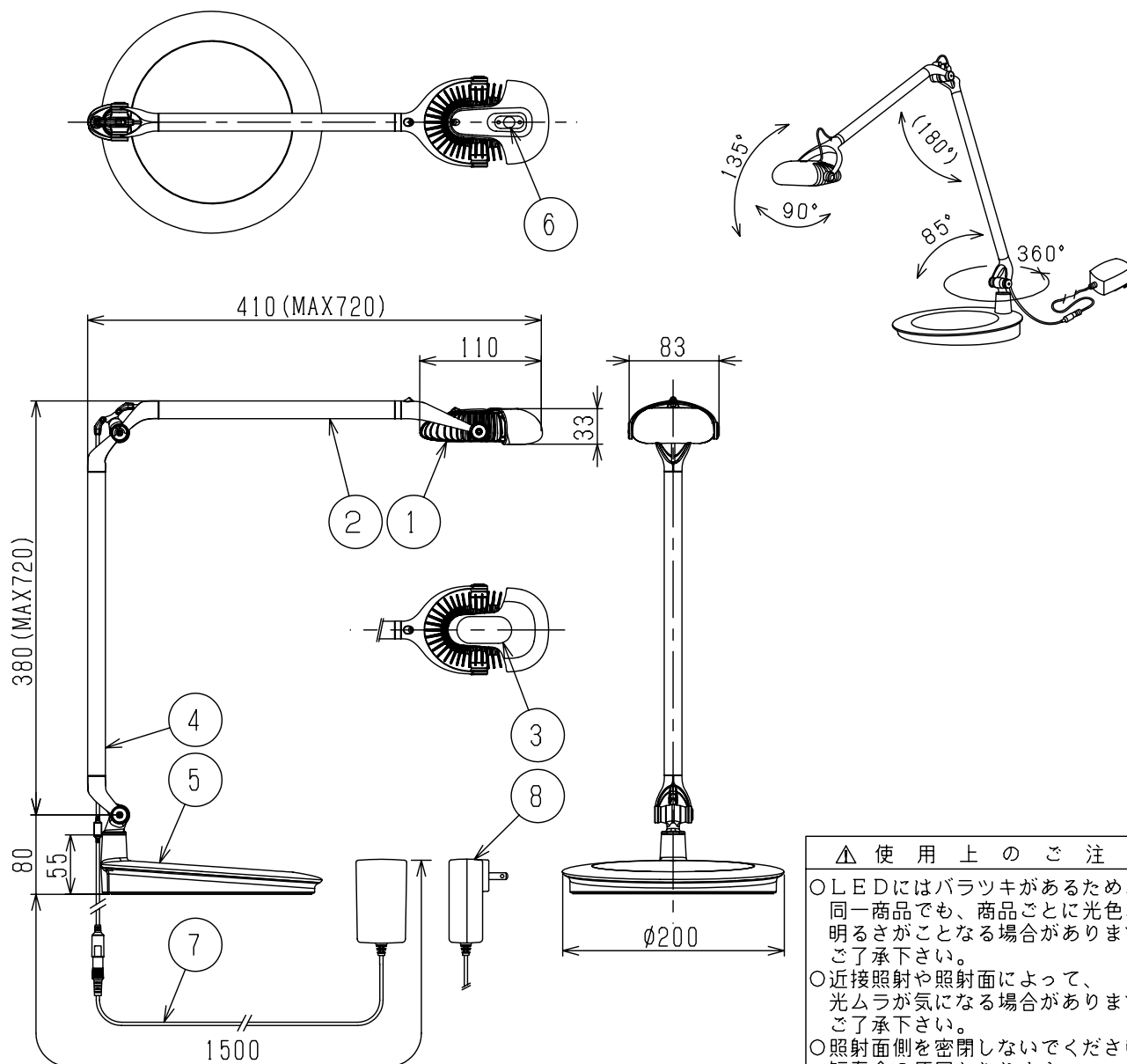
アーム・ヘッド可動範囲図
