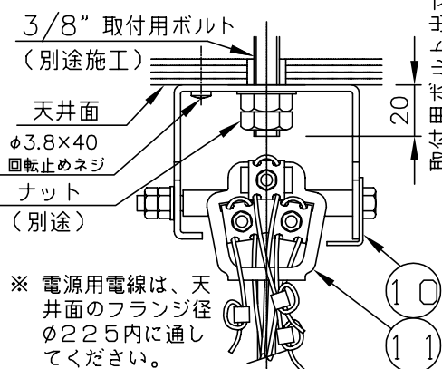
天井取付部詳細図
