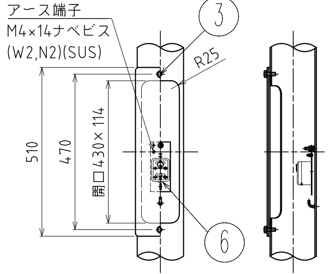
開口部詳細
