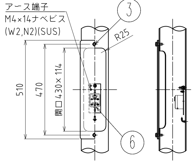
開口部詳細
