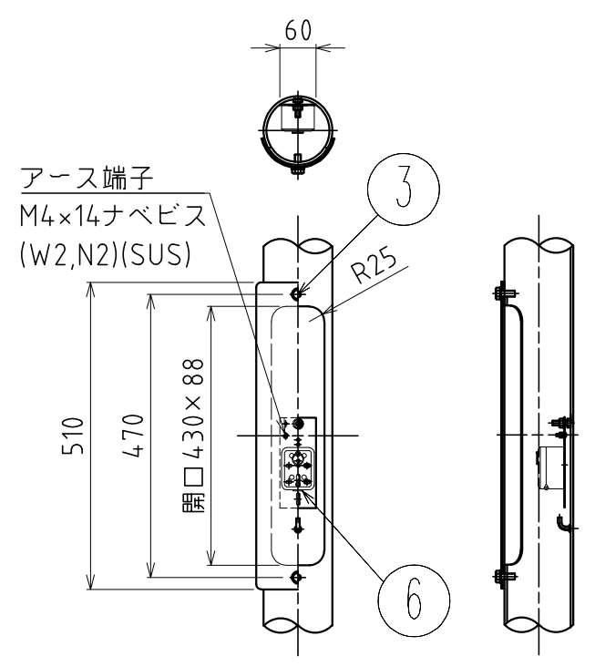
開口部詳細
