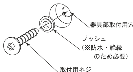
図 3 取付ネジの注意
