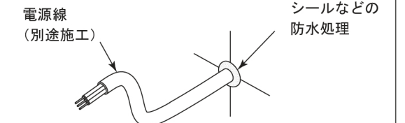
図 4 電源線入り口の処理
