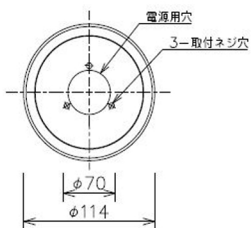
■ 図-1 ■ 取付ピッチ
