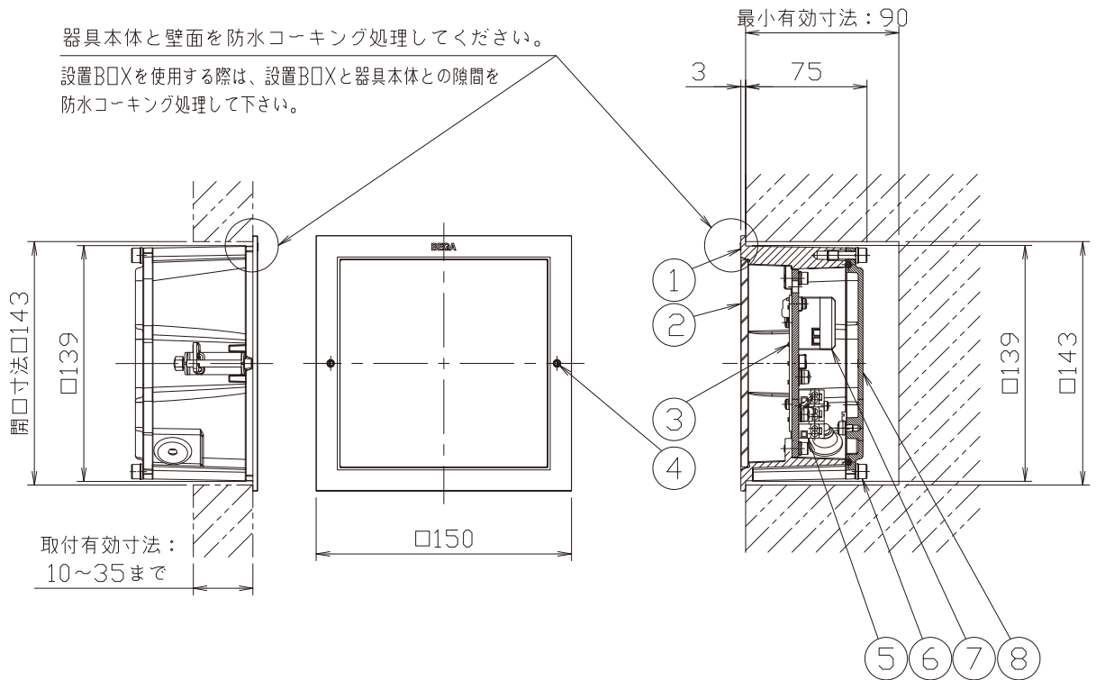
切込寸法
