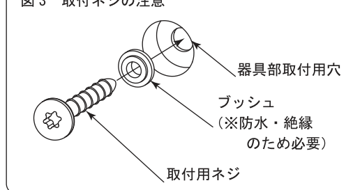
図3 取付ネジの注意
