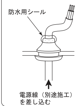
図7 電源線防水処理
