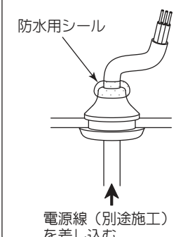
図8 電源線防水処理
