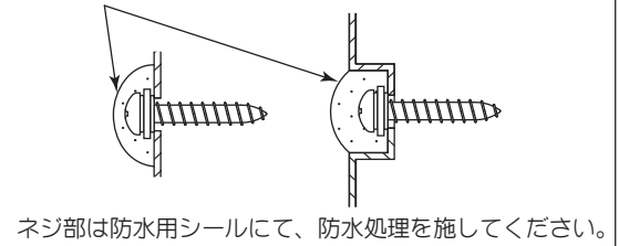
図6 防水用シールなどの防水処理
