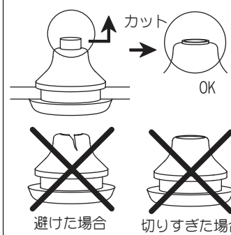
図7 グロメット処理方法
