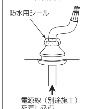
図 7 電源線防水処理
