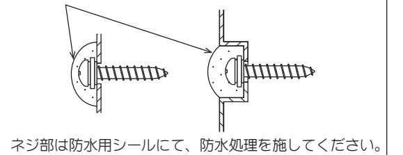
図5 防水用シールなどの防水処理
