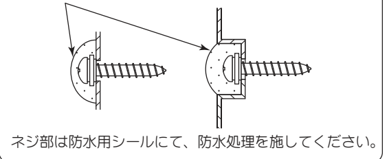
図6 グロメット処理方法
