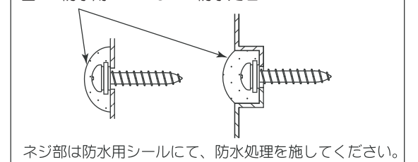
図3 グロメット処理方法
