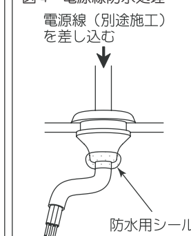
図4 電源線防水処理
