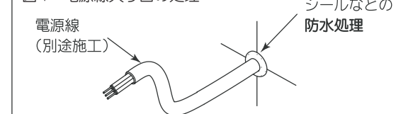
図1 電源線入り口の処理
