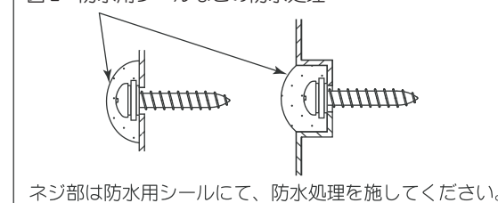
図2 防水用シールなどの防水処理
