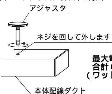
<図1> アジャスタ取り外し方法
