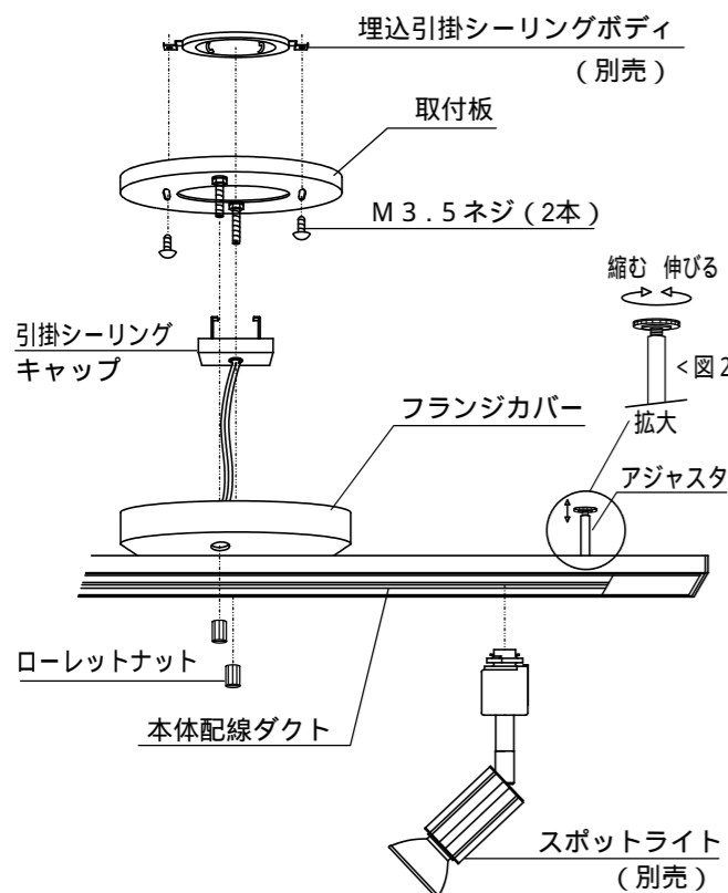
<図1> アジャスタ取り外し方法
