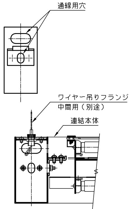
連結部詳細図
