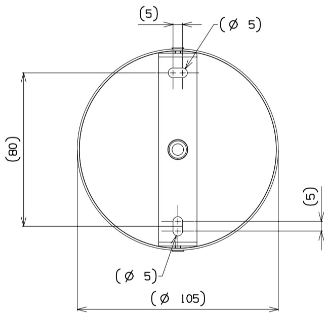
Detail systeme de fixation Ech 1:2
