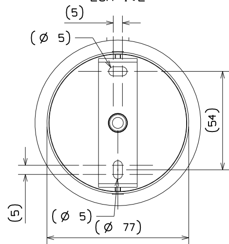
Detail systeme de fixation Ech 1:2
