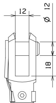
DETAIL BELIERE ECHELLE 1:2
