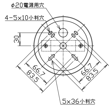
取付部詳細
