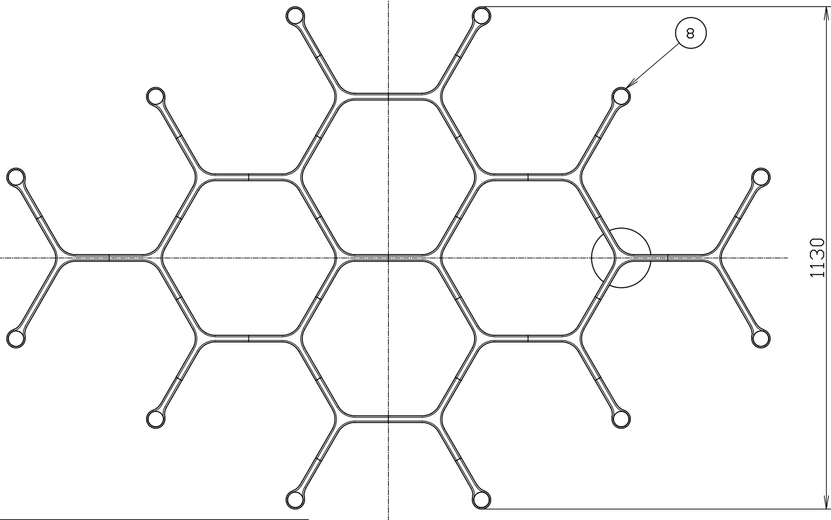
取付寸法 (天井伏図)
