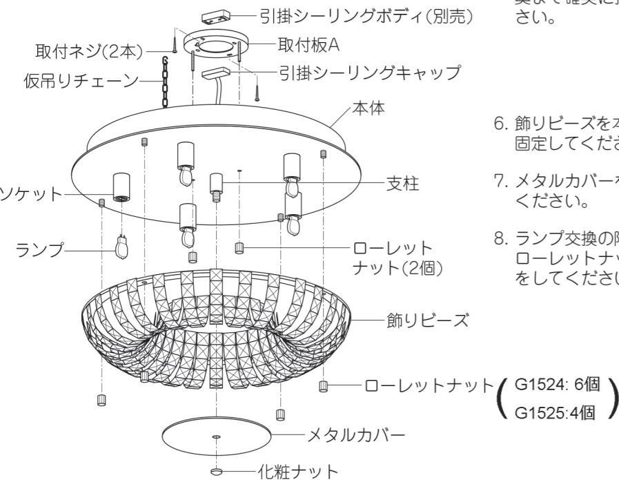
[図1-a 角形・丸型引掛シーリングの場合]
