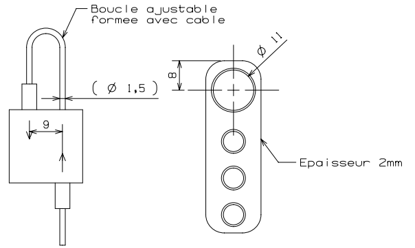
Detail system de fixation Ech 1:1
