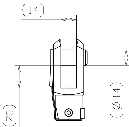
Detail Beliere Ech. 1:2
