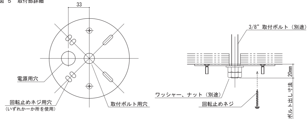
図 5 取付部詳細
