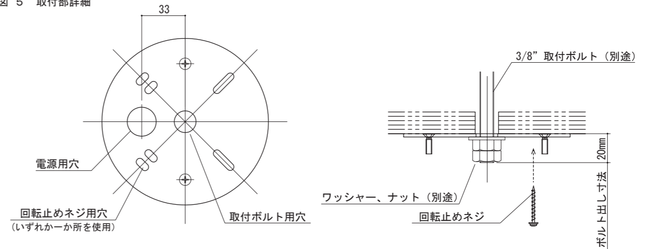
図 5 取付部詳細
