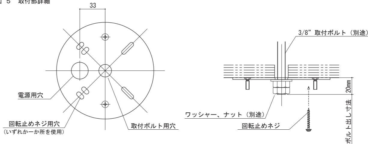
図 5 取付部詳細
