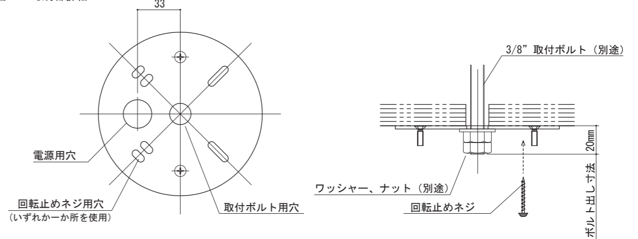
図 5 取付部詳細
