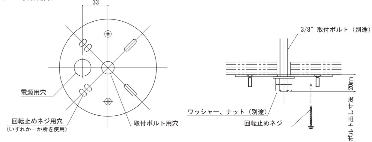
図 5 取付部詳細
