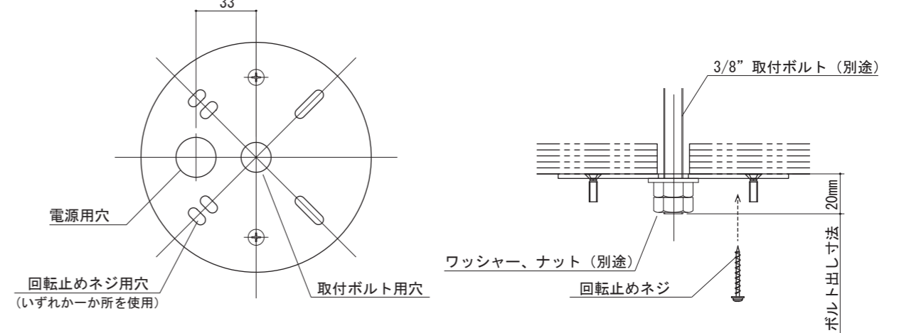
図 5 取付部詳細
