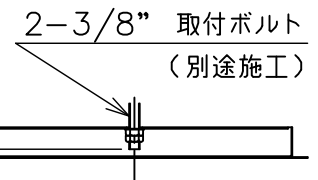
取付部詳細
